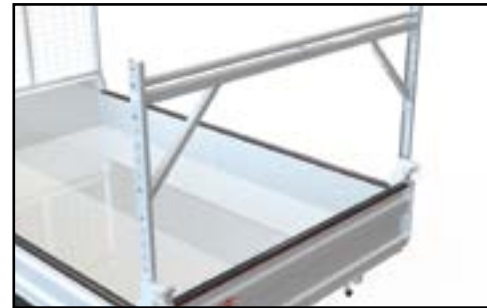
Porte-madrier avec rouleaux - hauteur ajustable
